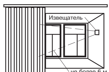
Рисунок 8 – Установка извещателя между стеклом и занавесями (балкон)
